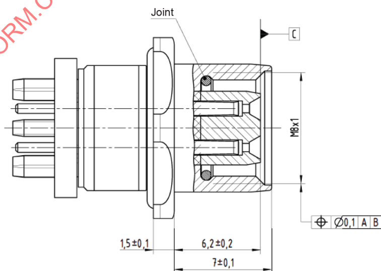
Figure 13 – Dimensions d'accouplement du modèle 6J-M8
