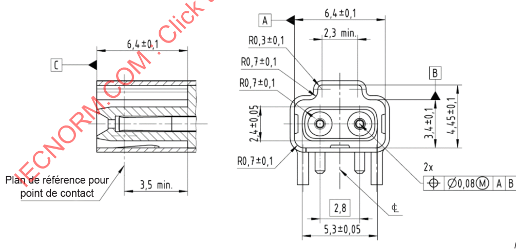
Figure 3 – Dimensions d'accouplement du modèle 2J-L
