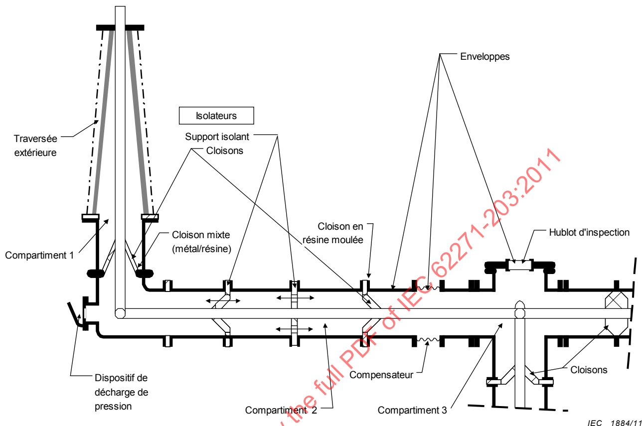
Figure 2 – Exemple de disposition des enveloppes et des compartiments à gaz
