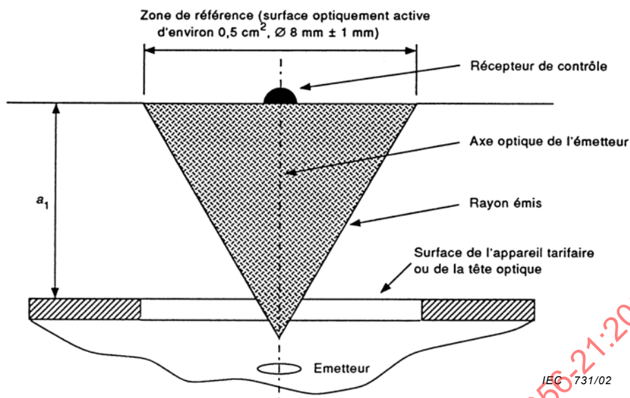
Figure 5 – Disposition d'essai pour l'émetteur
