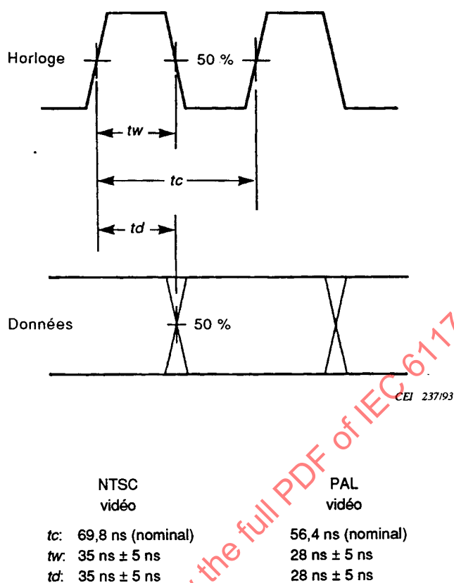
Figure 48 – Forme d'onde d'horloge de l'interface parallèle vidéo numérique
