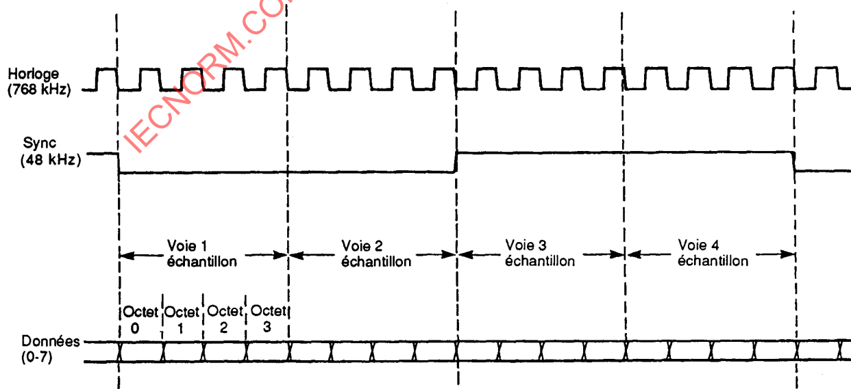
Figure 51 – Synchronisation de l'interface parallèle audionumérique
