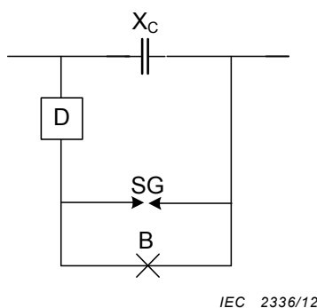
2a) Éclateur simple (type K1)
