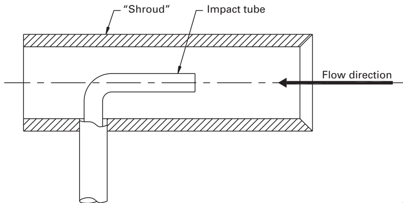
Fig. 5-2.1.2-1 Keil Probe
